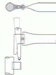
Rail-to-frame wedgeloc connection
